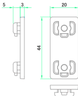
フック 部品
