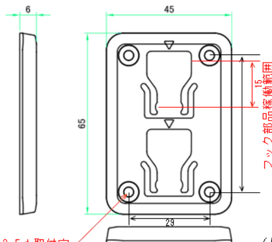
ベース 部品
